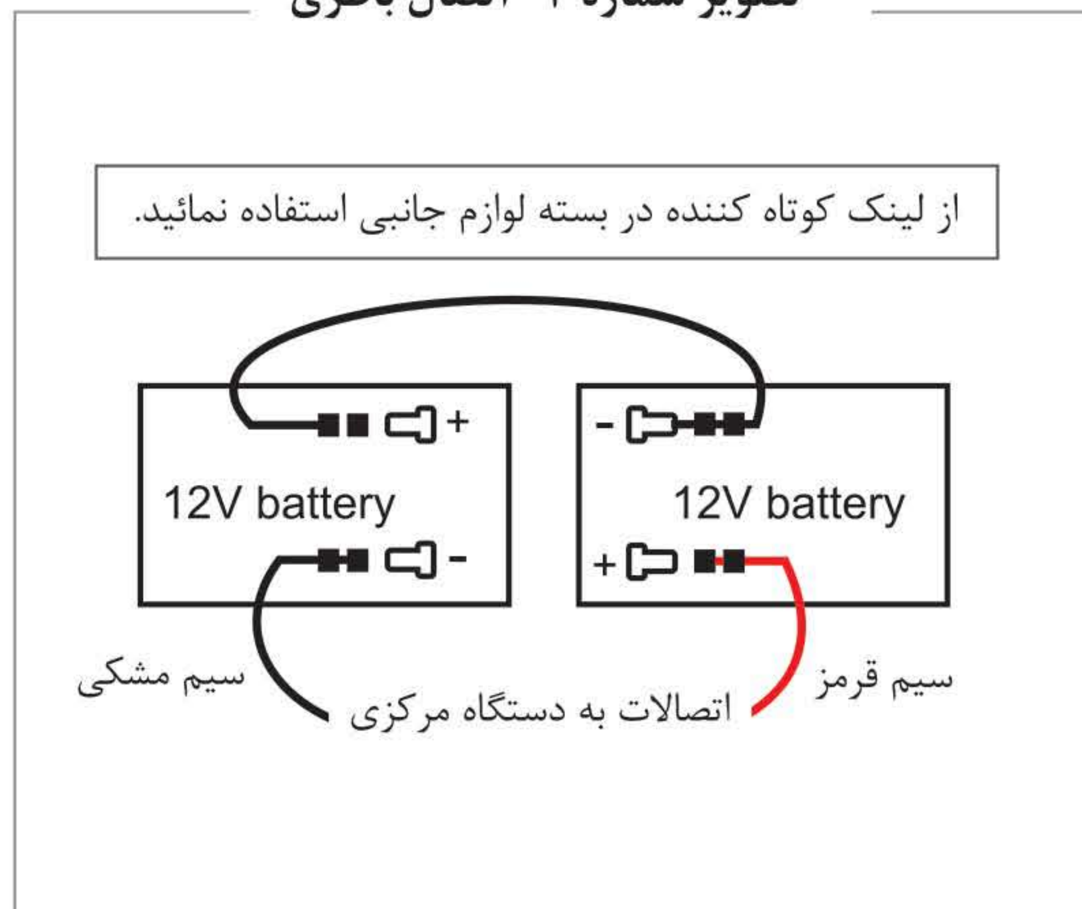
تصویر شماره ۲- اتصال باتری
